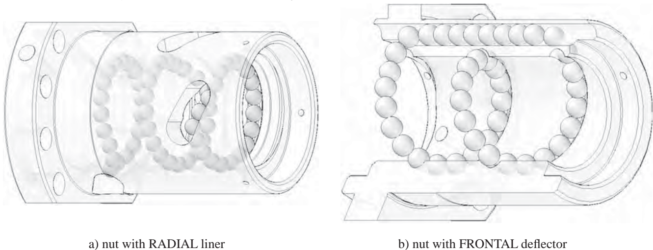
Fig. 3 - Ball recirculation
